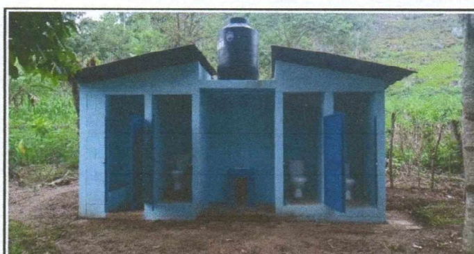
Foto 6: CULMINACION DE SUSTITUCION DE INODOROS Y TINACO
